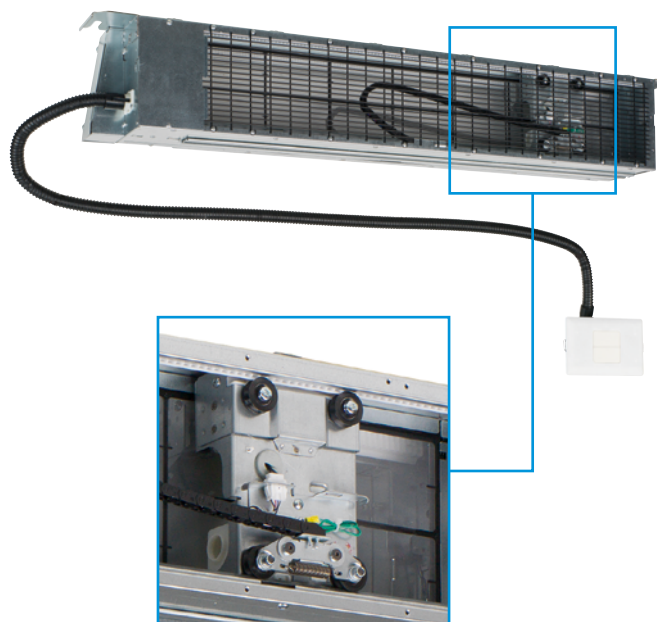
Optie voor zelfreinigende filter
