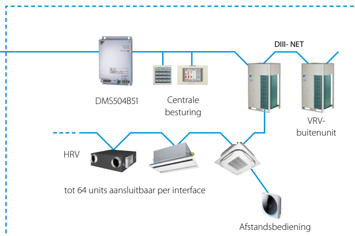
VRV-netwerk
