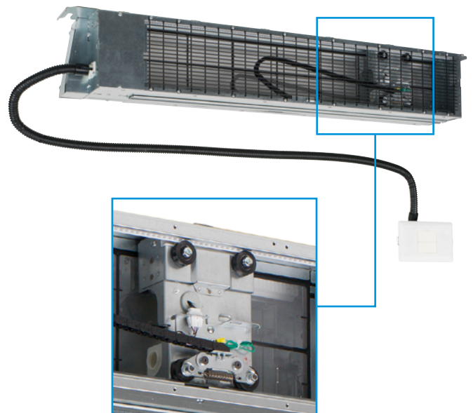
Optie voor zelfreinigende filter
