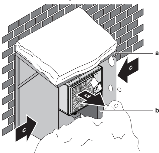
a Afdakje tegen de sneeuw b Voetstuk (minimale hoogte=150 mm) c Belangrijkste windrichting d Luchtuitlaat
