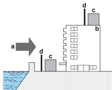
a Zeewind b Gebouw c Buitenunit d Afscherming tegen wind
