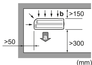
a Luchtuitlaat b Luchtinlaat
