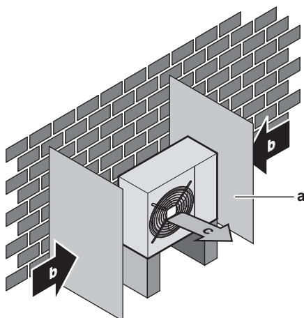
a Geleideplaat b Belangrijkste windrichting c Luchtuitlaat
