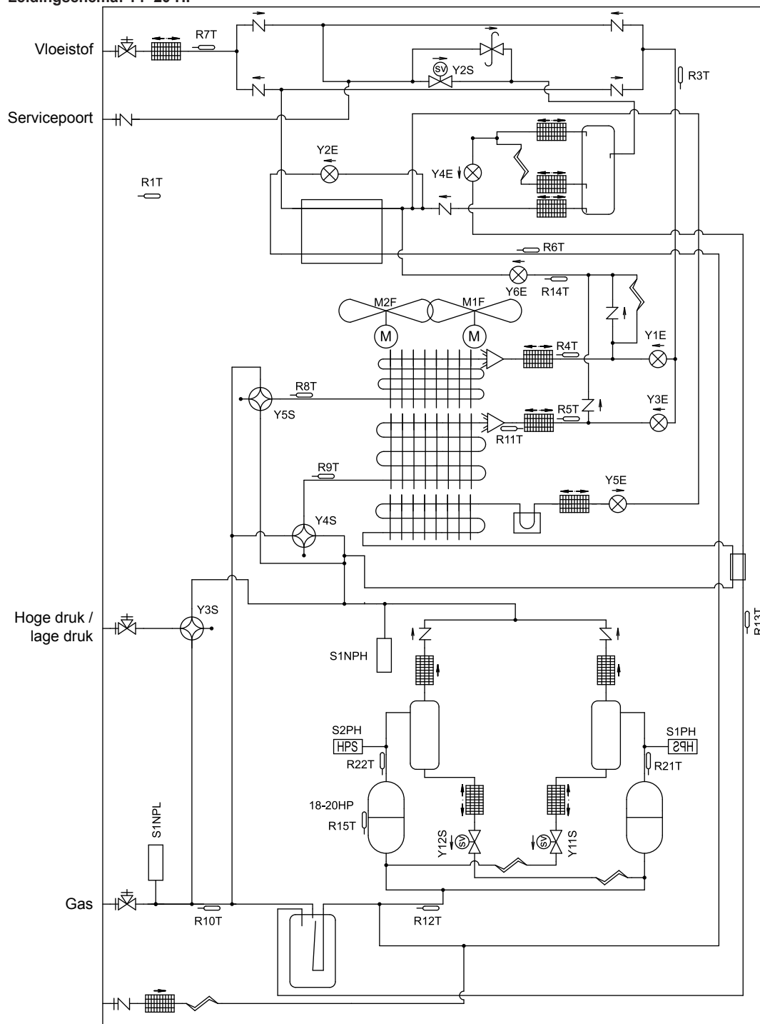
Leidingschema: 14~20 HP
