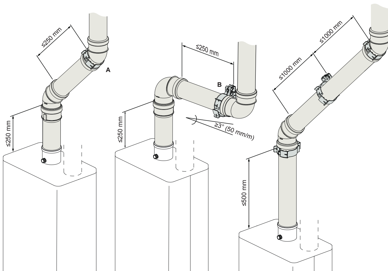
A Tweede klem na het tweede bochtstuk B Eerste klem na het tweede bochtstuk
