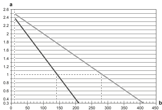
a Voordruk (bar) b Maximum watervolume (l) — Maximum aanvoerwatertemperatuur van 55°C voor vloerverwarmingstoepassingen - - - Maximum aanvoerwatertemperatuur van 80°C voor radiatortoepassingen
