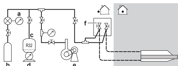
a Manometer b Stikstof c Koelmiddel d Weegschaal e Vacuümpomp f Afsluiter
