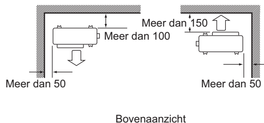
Muren aan drie kanten
