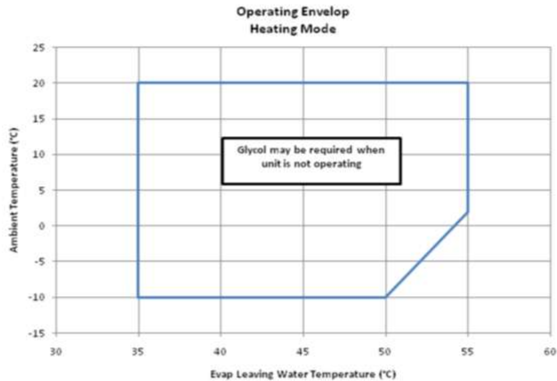
Illustration 2 – Limites opérationnelles en mode de chauffage - EWYD~BZSS / EWYD~BZSL
