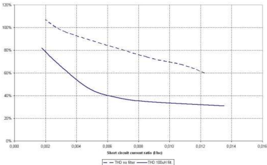
Illustration 18 – Teneur en harmoniques avec et sans inductance de ligne
