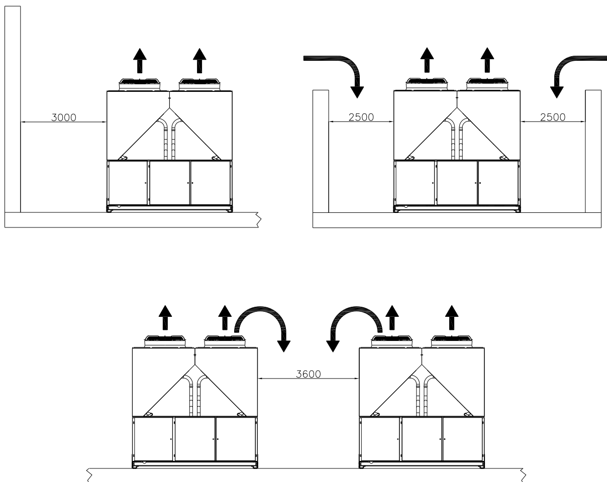
Illustration 5 - Dégagement minimum recommandé pour l'installation
