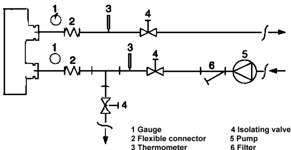
Illustration 6 – Raccordement du tuyau d'eau de l'évaporateur
