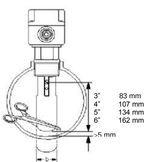
Illustration 8 - Ajustement du contacteur de débit de sécurité
