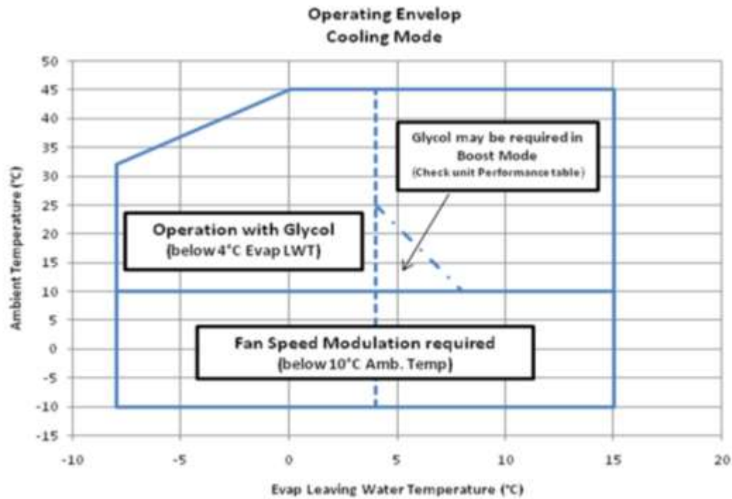
Illustration 1 – Limites opérationnelles en mode de refroidissement - EWYD~BZSS / EWYD~BZSL
