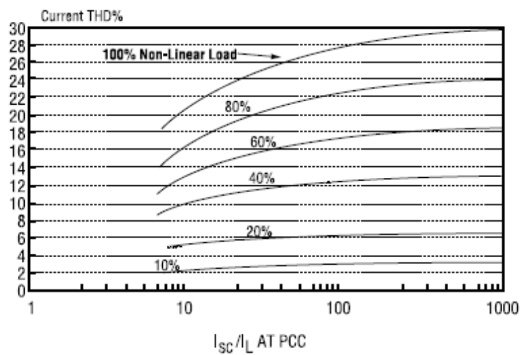
Illustration 19 – Teneur en harmonique variant en fonction du pourcentage de charges non linéaires
