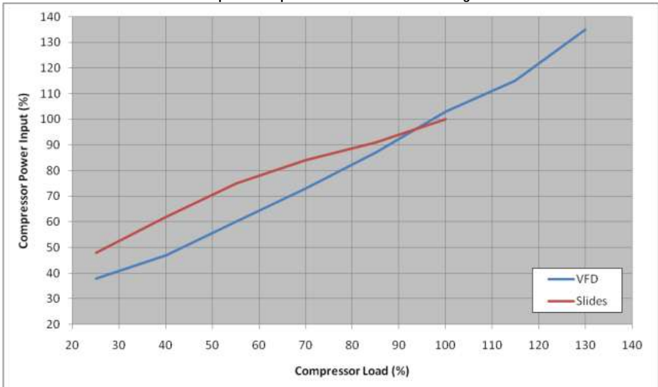
Illustration 15 – Puissance absorbée par le compresseur en fonction de la charge
