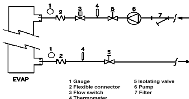
Illustration 6 – Raccordement du tuyau d'eau de l'évaporateur
