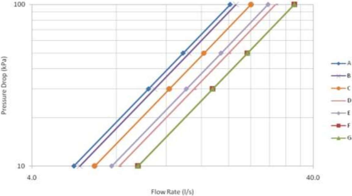
Illustration 12 – Chute de pression d’évaporateur
