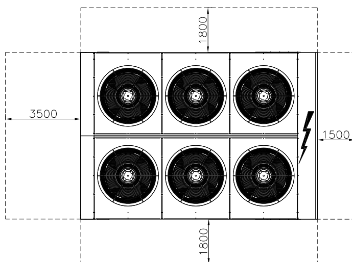
Illustration 4 - Exigences de dégagement minimum pour l'entretien de la machine
