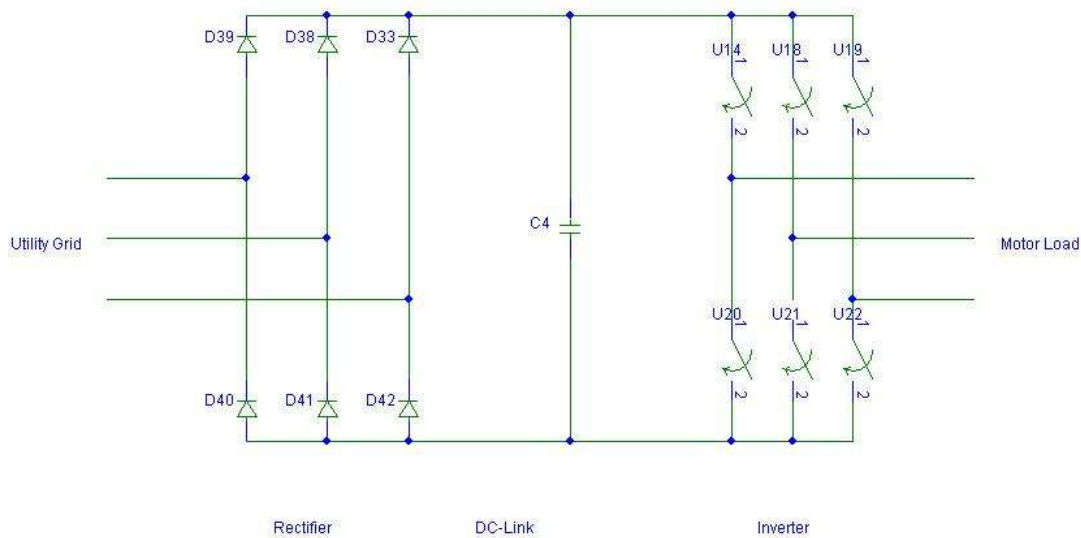
Illustration 16 – Schéma typique d'un VFD
