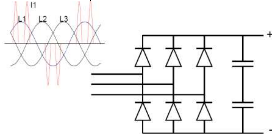
Illustration 17 – Harmoniques sur le réseau
