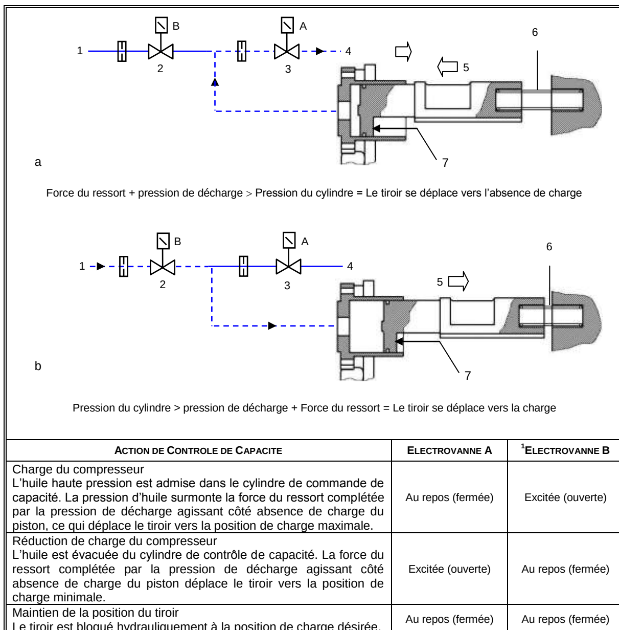
Illustration 25 - Contrôle de capacité variable en continu pour le compresseur Fr3100
