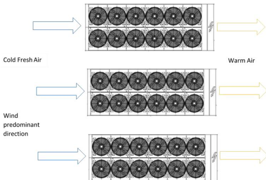
Fig. 4 - Installatie meerdere systemen (modus koeling)
