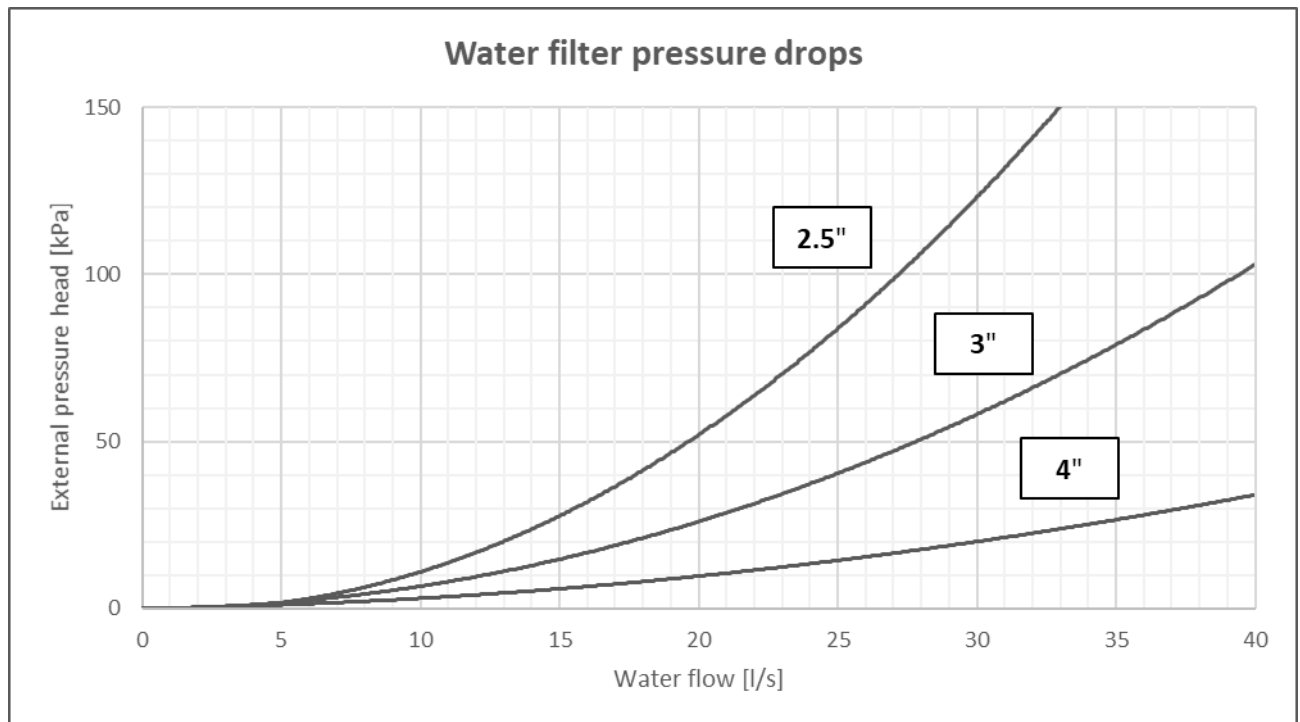
Afb. 5 - Drukvermindering waterfilter
