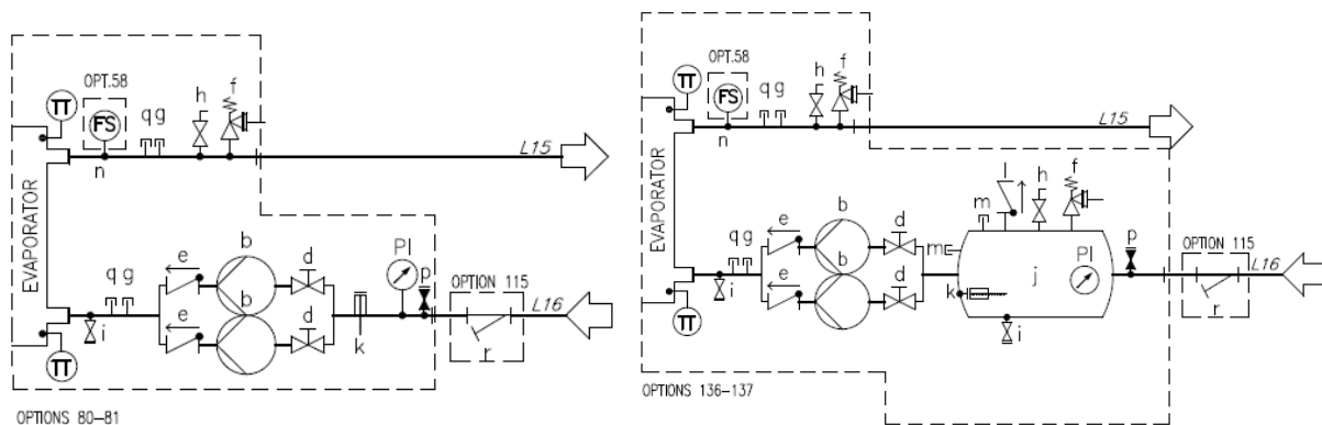
Afb. 9 - Hydraulisch schema voor dubbele pomp (EWYTx5B) (optie 80-81/136-137) (max. bedrijfsdruk 6 bar)
