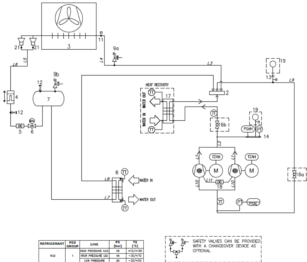
Afb. 17 - Systeem met enkel circuit EWYTx5B schema koelleidingen (P&ID)
