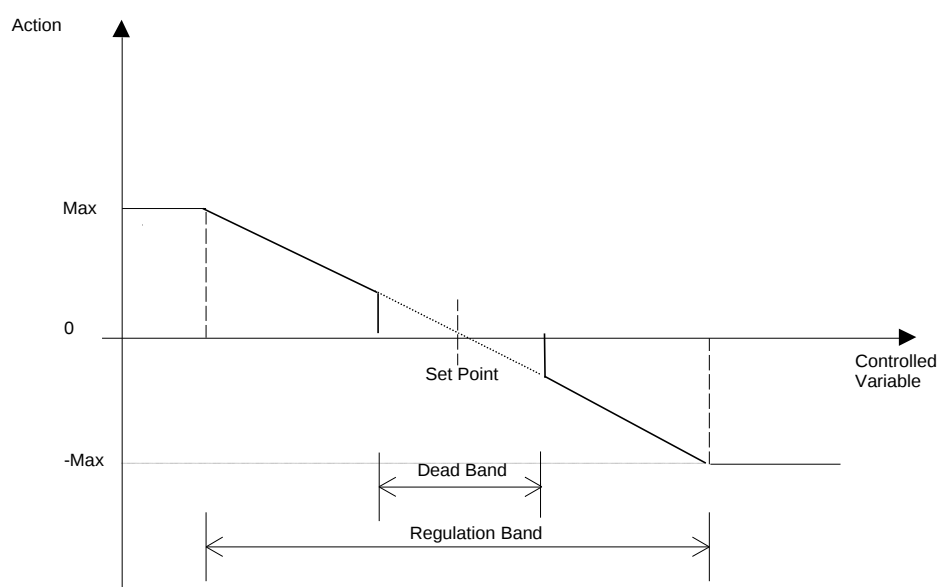
Figure 16 – Action proportionnelle du PID VSD en mode chauffage
