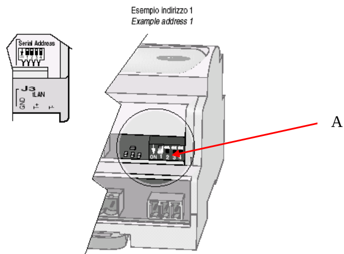
A. Commutateurs d'adressage
