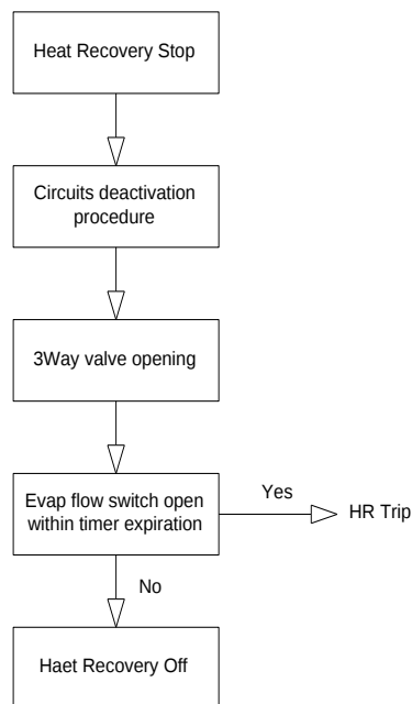
Figure 20 – Séquence d’arrêt de la récupération de chaleur
